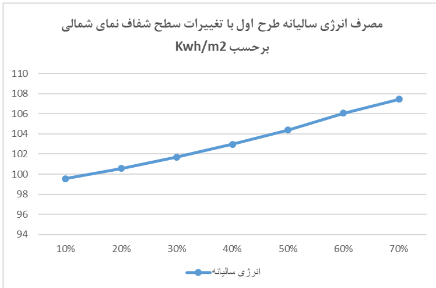
شکل ۴. میزان انرژی کل مصرفی در ساختمان‌های طرح اول
