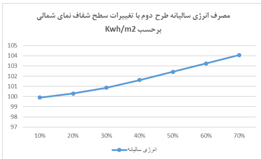
شکل ۱۵. میزان انرژی کل مصرفی در ساختمان‌های طرح دوم دارای ۱۰ درصد سطح شفاف در نمای جنوبی، با تغییر سطح شفاف نمای شمالی
