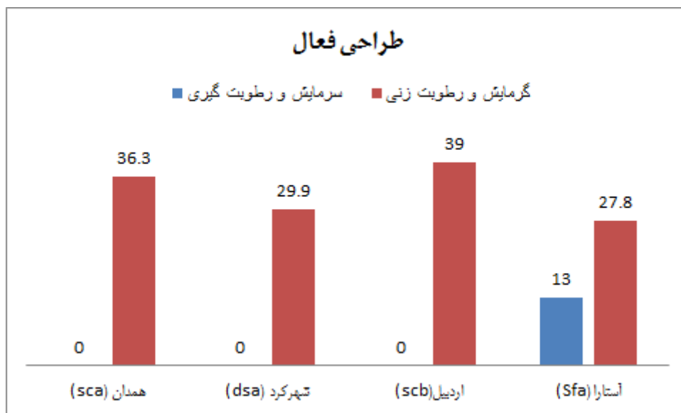
شکل ۱۰. استراتژی طراحی فعال بر حسب درصد
