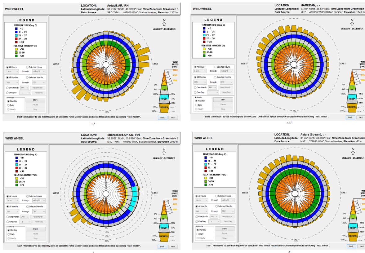
شکل ۸. چرخ باد الف. همدان. ب. اردبیل. ج. آستارا. د. شهرکرد (مرجع: نرم افزار کلایمت کانسلانت)
