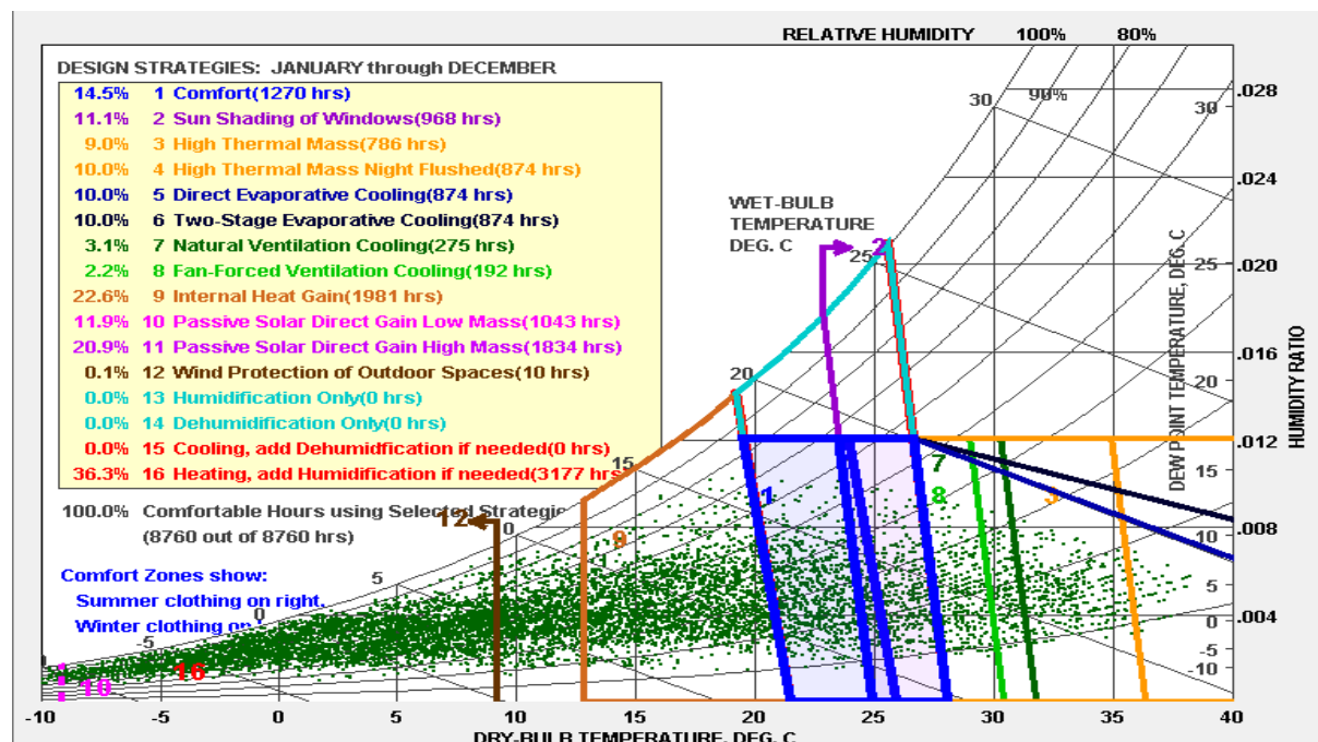
شکل ۹. چارت سایکرومتریک همدان (مرج: نرم افزار کلایمت کانسلانت)
