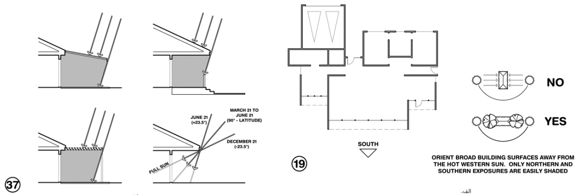
شکل ۱۲. تدبیر معماری الف) جهت قرارگیری پنجره ها ب) طراحی سایبان (مرجع: نرم افزار کلایمت کانسلانت)
