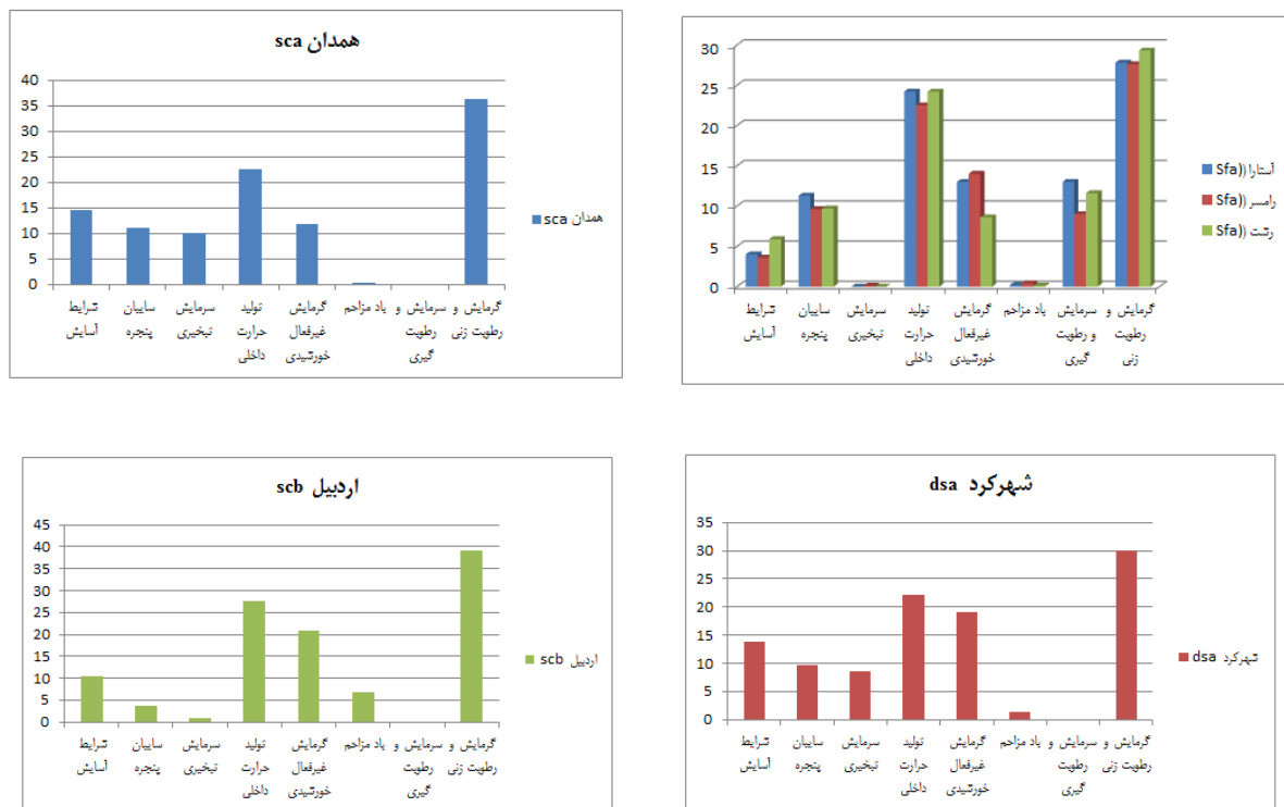
شکل ۱۴. نمودار مقایسه ای اقلیم های Sca, Sfa, Scb و Dsa
