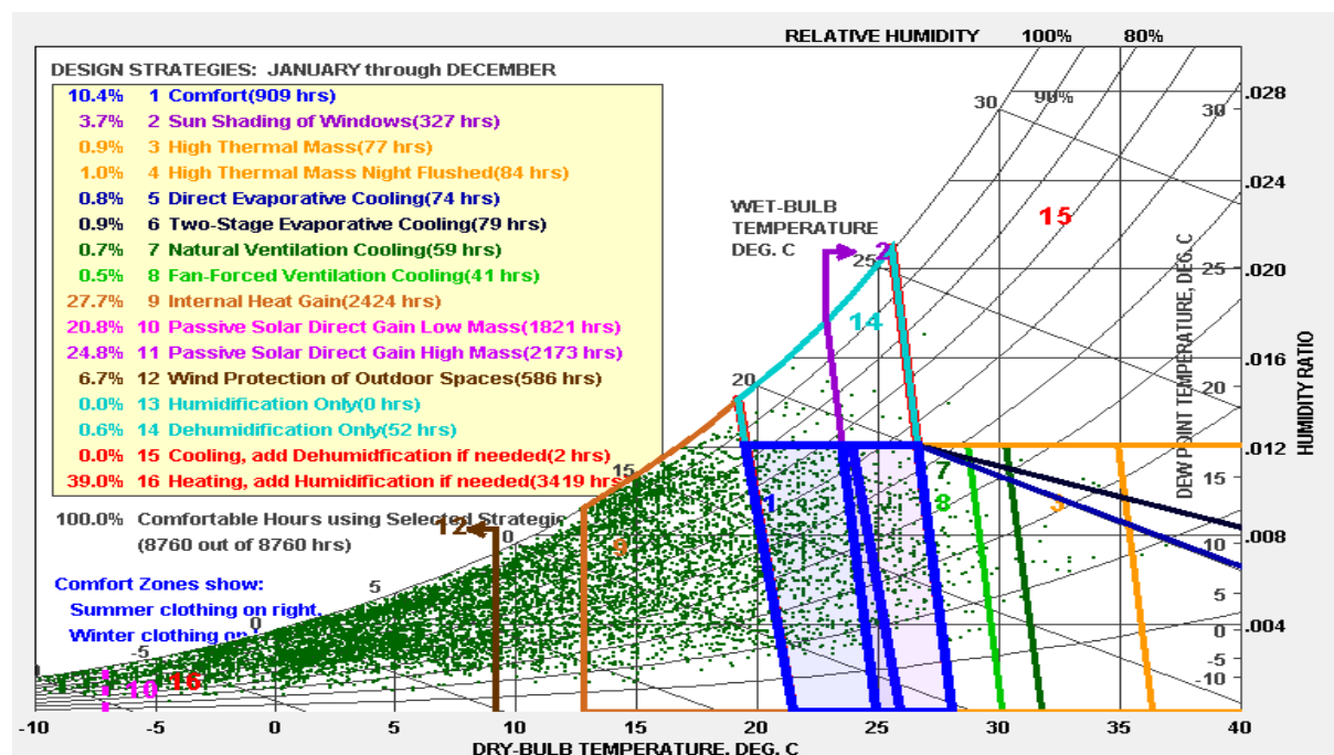
ادامه شکل ۹. چارت سایکرومتریک اردبیل
