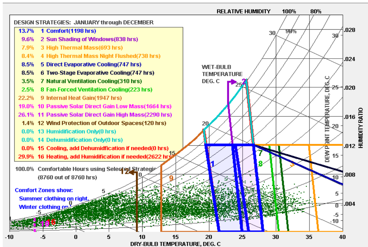
ادامه شکل ۹. چارت سایکرومتریک شهرکرد
