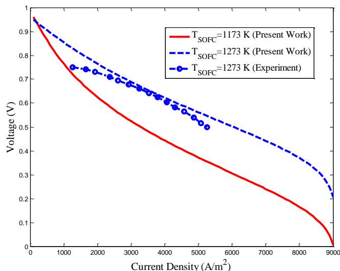
شکل ۴. نمودار ولتاژ پیل سوختی بر حسب چگالی جریان و مقایسه با مقدار تجربی [۱۴] در دمای ۱۲۷۳ کلون
