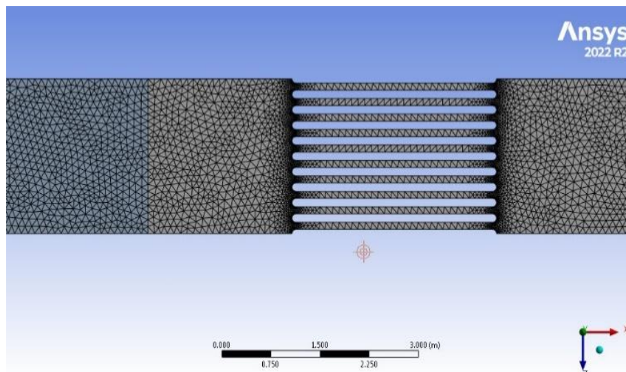
شکل ۷. شبکه درشت
