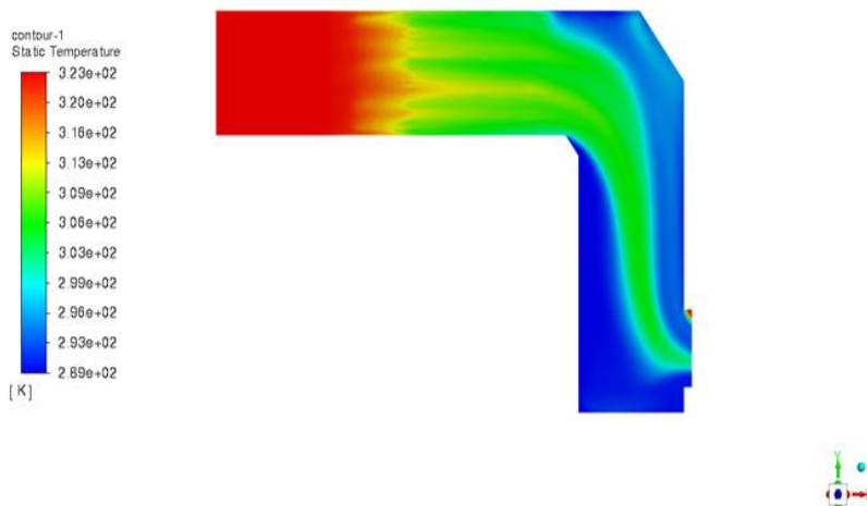
شکل ۱۹. کانتور دما
