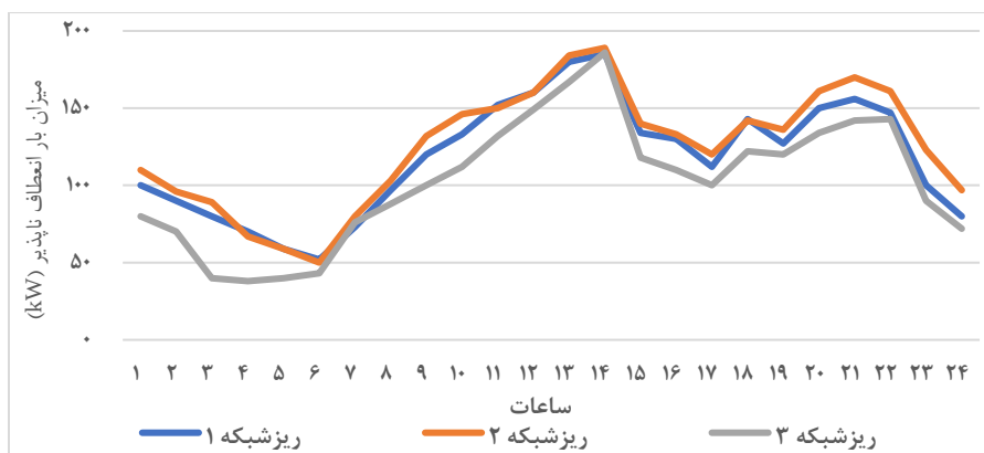
شکل ۷ میزان بار انعطاف پذیر در سیستم ریشبکه چندگانه
