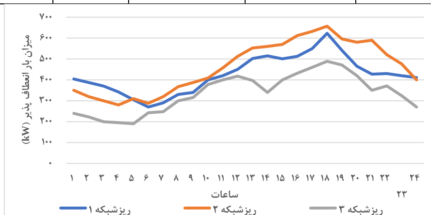
شکل ۶ میزان بار انعطاف پذیر در سیستم ریشبکه چندگانه.
