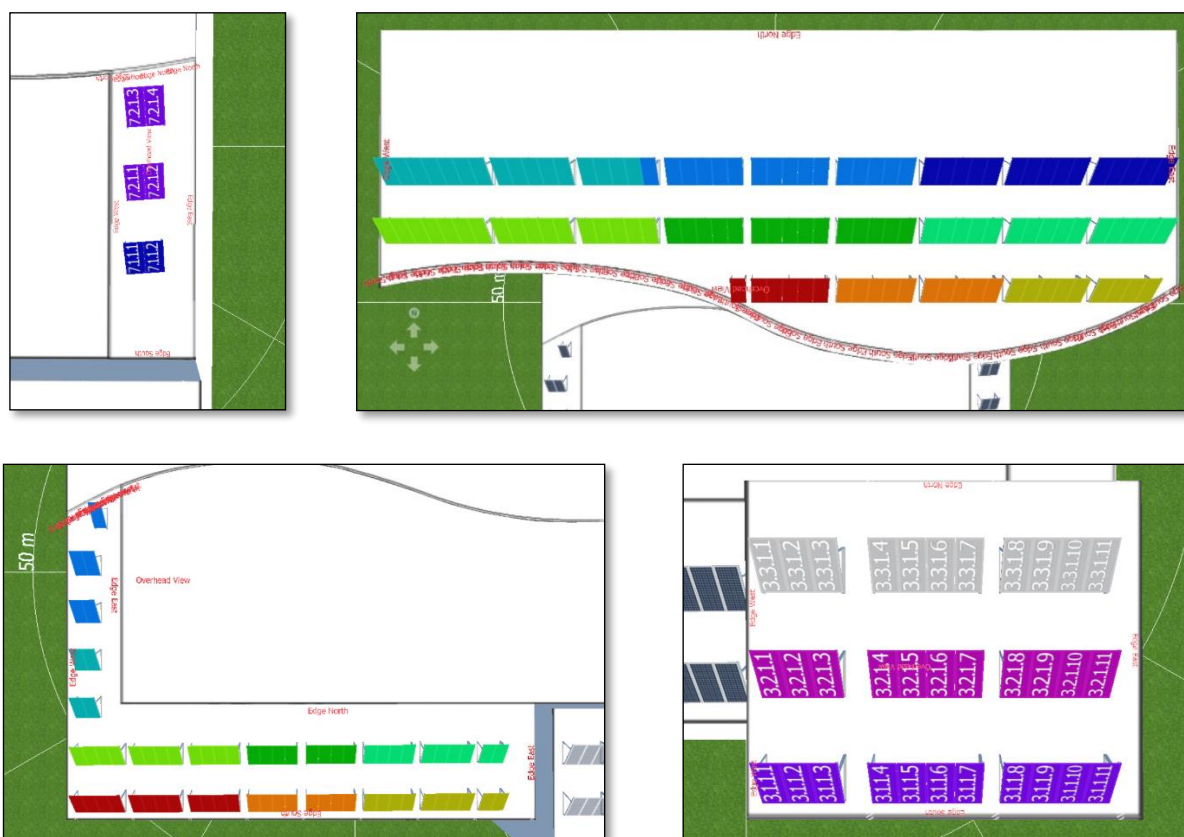
شکل ۷. اتصالات الکتریکی و آرایش استرینگ‌ها به اینورترها
