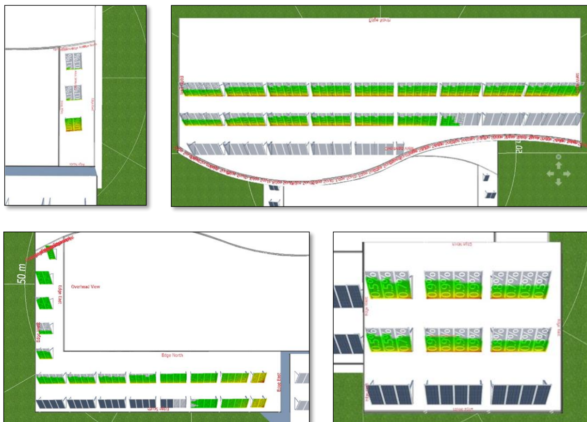
شکل ۶. درصد سایه‌اندازی بر پنل‌ها در بخش‌های مختلف بام
