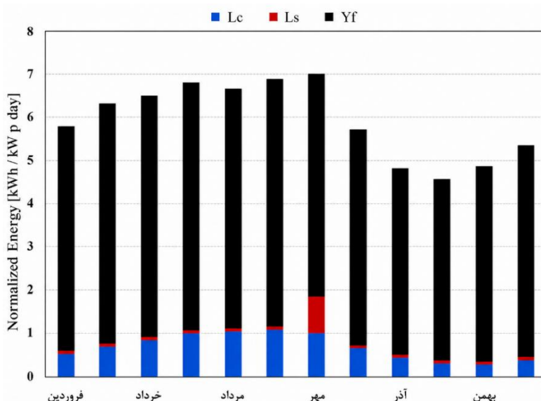
شکل ۴. انرژی و تلفات تولید شده سامانه فتوولتاییک
