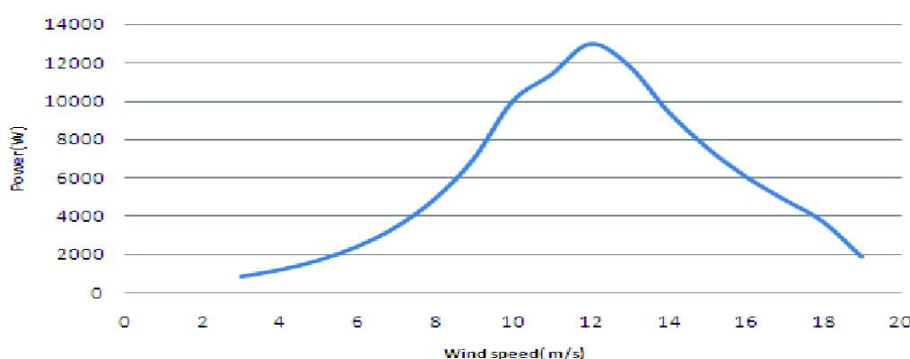
شکل ۲: منحنی انرژی توربین بادی مدل FD8.0-10K-20 [۴]
