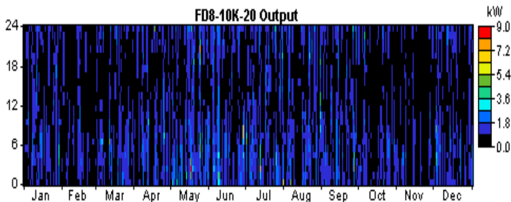
شکل ۱۲: میزان انرژی تولید شده از توربین بادی در یک سال
