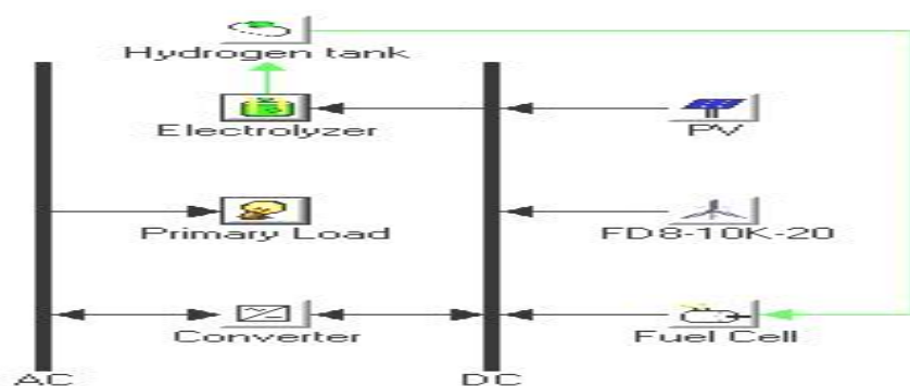
شکل ۷: نمایی شماتیک از طرح سیستم هیبرید فتوولتائیک/باد با ذخیره هیدروژن در سایت طالقان در نرم‌افزار HOMER
