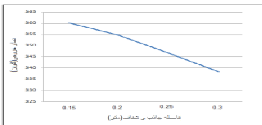
شکل ۴) بررسی اثر فاصله سطح شفاف و جاذب
