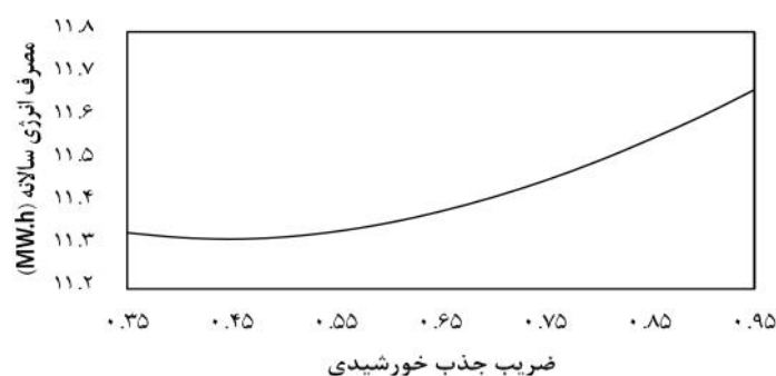
شکل ۷) نمودار مصرف سالانه انرژی به ازای ضرایب جذب مختلف برای یک نما در شهر تهران
