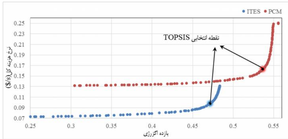
شکل ۴) منحنی بهینه سازی Pareto Front برای دو سیستم PCM و ITES
