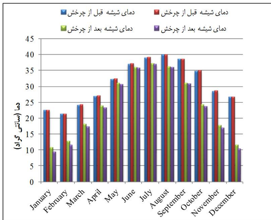
شکل ۱۱. مقایسه نمای شیشه‌ای در حالت موجود با حالت چرخش ۱۸۰ درجه‌ای
