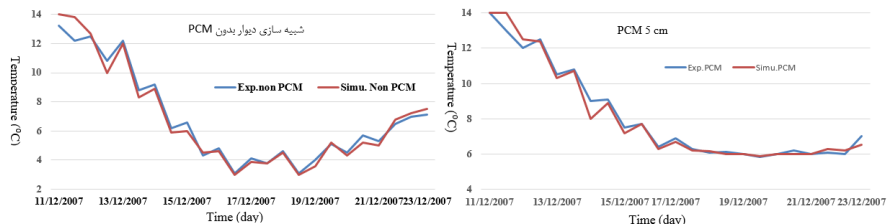
شکل ۶. مقایسه‌ی نتایج تجربی (پسوپاتی، ۲۰۰۸) و شبیه‌سازی دمای داخلی دیوار
