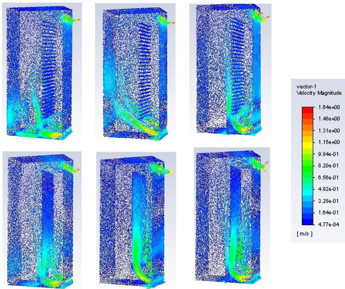
شکل ۶- جریان هوا در حفره میانی نمای دوپوسته - عرض حفره ۷۵ سانتیمتر و زاویه سایه بان صفر درجه (تصاویر بالا) و ۹۰ درجه (تصاویر پایین) و از راست به چپ سطح مقطع دریچه ها ۰،۱۰، ۰،۲۰ و ۰،۳۰ متر مربع خروجی نرم افزار فلوئنت
