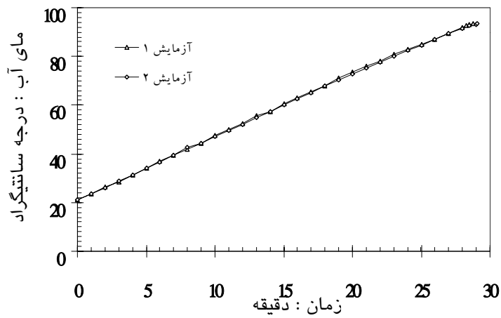
نمودار ۱- زمان جوش آمدن آب به میزان ۵۴۰۰ سانتیمتر مکعب در سماور برقی ۶ لیتری خانگی
