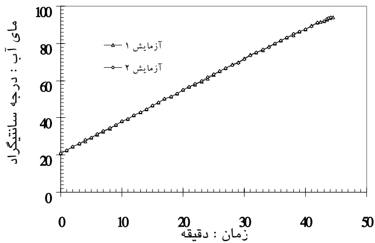
نمودار ۲- زمان جوش آمدن آب به میزان ۱۸۰۰۰ سانتیمتر مکعب در سماور برقی ۳۰ لیتری تجاری
