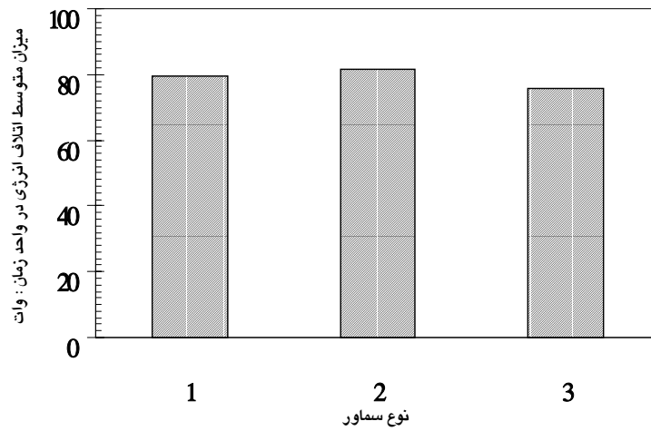
نمودار ۴- میزان اتلاف انرژی در واحد زمان در سماورهای برقی ۳۰ لیتر تجاری
