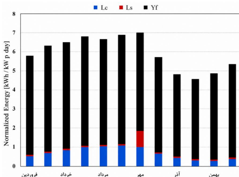
شکل ۴. انرژی و تلفات تولید شده سامانه فتوولتاییک
