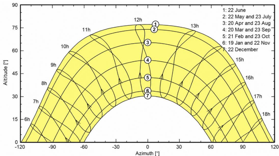
شکل ۳. مسیر خورشید در سد طالقان (نرم‌افزار PVSyst نسخه ۷.۰)
