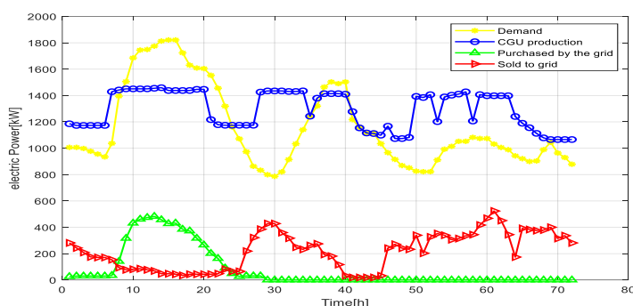
شکل ۲ خروجی توان الکتریکی شبیه سازی شده در سیستم بدون ذخیره ساز UPS و باتری های لیتیومی
