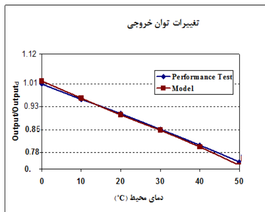
شکل ۱۰: نمودار تغییرات توان خروجی سبیل بر حسب دمای محیط و مقایسه با شرایط واقعی
