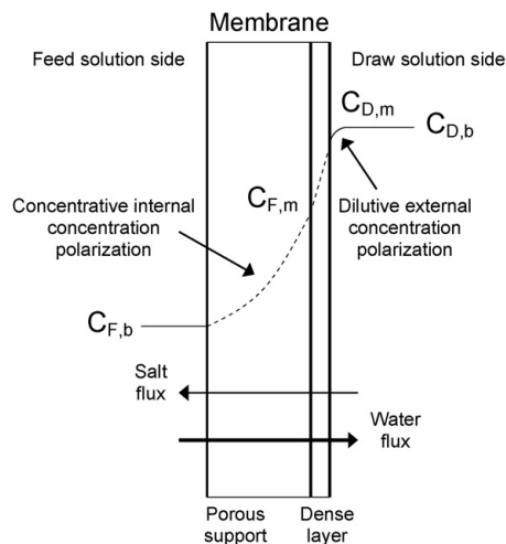
شکل ۸: نمایش یک غشای نامتقارن در روش PRO با قطبش غلظت داخلی و خارجی و نمایش جهت جریان و نمک
