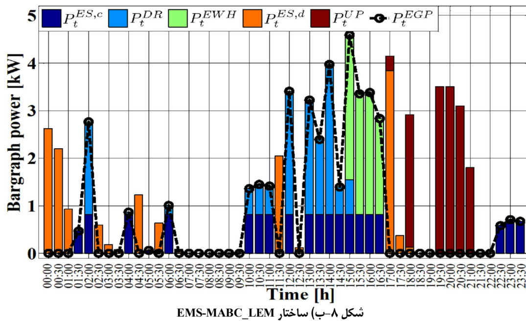
شکل ۸) بارگراف مربوط به توان‌های بارهای غیرقابل قطع، دشارژ باتری و UP در طول ۲۴ ساعته عملکرد سیستم
