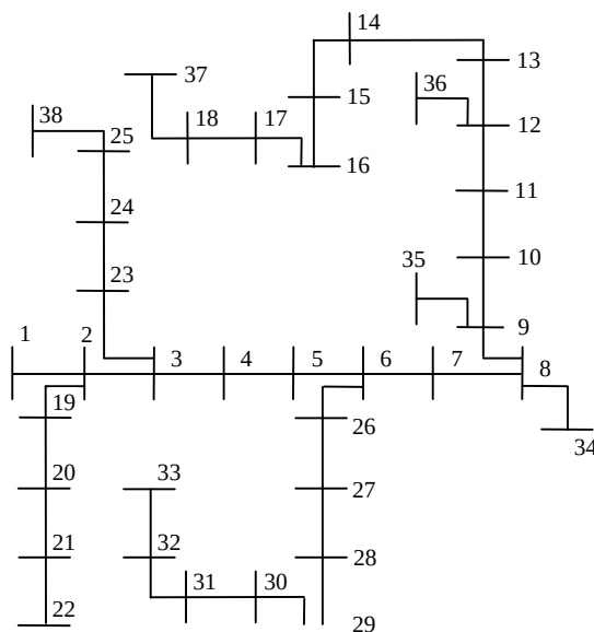
شکل ۳) شبکه توزیع ۳۸ شینه
