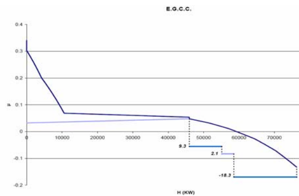
شکل ۲۹- دیاگرام EGCC
