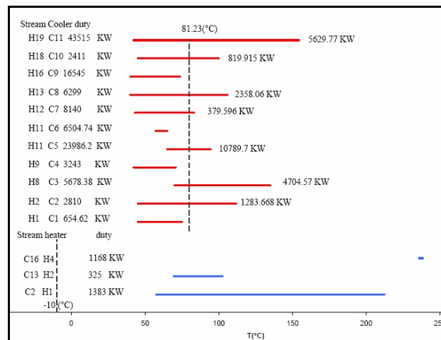
شکل ۲۳- بازه دمایی هیترها و کولرها
