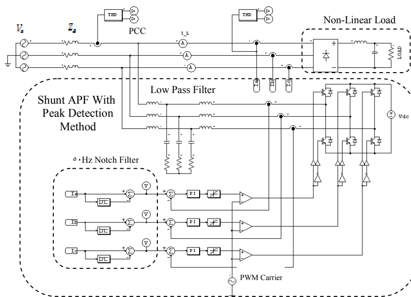
شکل ۹) شبیه‌سازی مدار فیلتر فعال با روش کنترلی حذف مولفه اصلی جریان با فیلتر میان‌گذر
