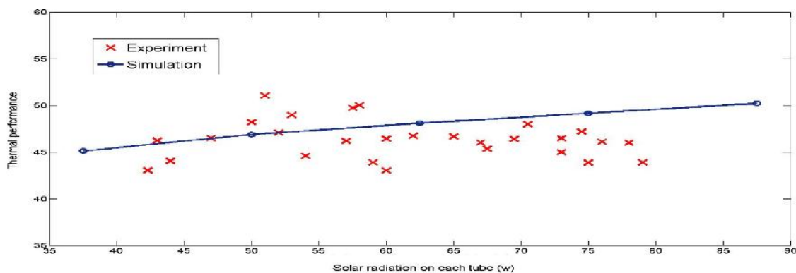
شکل ۱۱ بررسی تاثیر میانگین سطحی انرژی تابشی خورشید روی سطح لوله جاذب بر روی عملکرد حرارتی آنها
