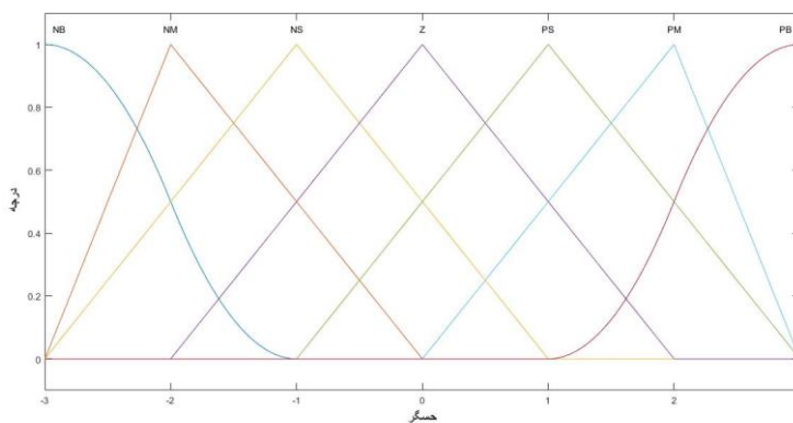
شکل ۷. ورودی حسگر و محرک فراز توربین بادی در کنترل کننده فازی
