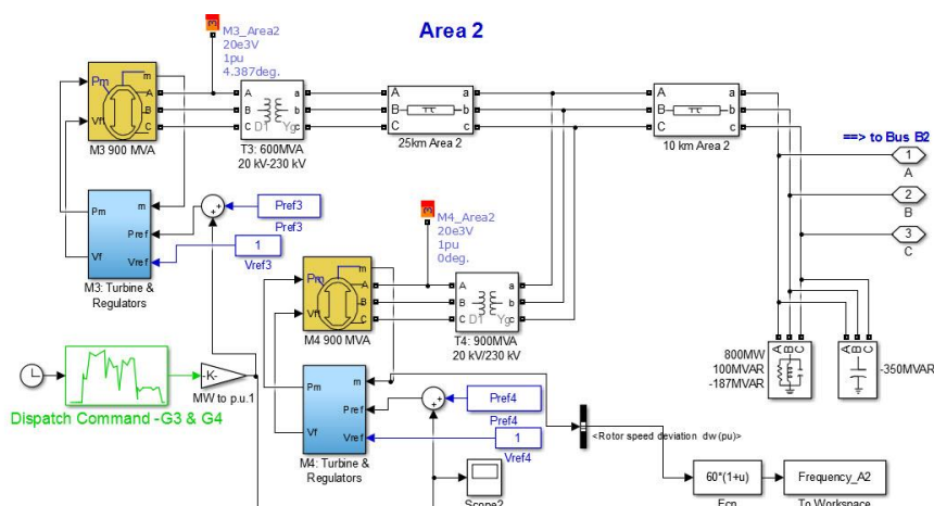
شکل ۱۳. نمای کلی سیمولینک طراحی شده برای سیستم ریزشکه متصل به توربین بادی
