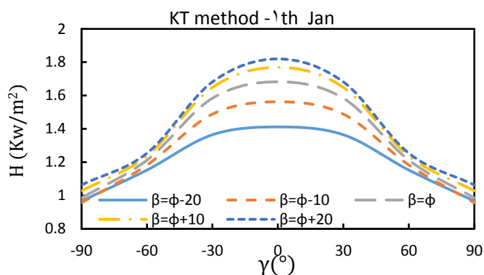
شکل ۷) مقادیر متوسط روزانه انرژی تشعشعی کل رسیده به یک سطح شیبدار بر حسب زاویه آزیموث مختلف برای زوایای مختلف شیبدار در اولین روز ماه ژانویه
