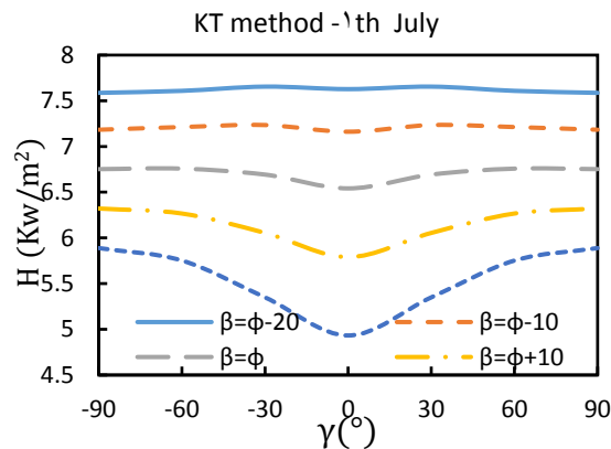
شکل ۹) مقادیر متوسط روزانه انرژی تشعشعی کل رسیده به یک سطح شیبدار بر حسب زاویه آزیموت مختلف برای زوایای مختلف شیبدار در اولین روز ماه ژوئیه.
