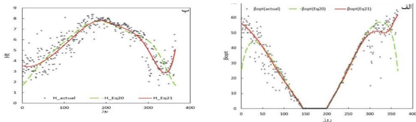
شکل ۵ (الف) زاویه شیب بهینه پنل بر حسب روزانه (ب) میزان H_t بدست آمده متناظر با \text{opt}\beta برای هر روز
