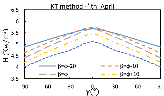
شکل ۸) مقادیر متوسط روزانه انرژی تشعشعی کل رسیده به یک سطح شیبدار بر حسب زاویه آزیموث مختلف برای زوایای مختلف شیبدار در اولین روز ماه آوریل.
