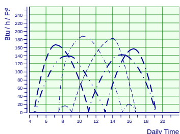
نمودار (۸) سطوح قائم (امتداد از جنوب 15°W) نمودار (۹) سطوح قائم (امتداد از جنوب 30°W) نمودار (۱۰) سطوح قائم (امتداد از جنوب 45°W) (بیگیری، ۱۳۹۹) (بیگیری، ۱۳۹۹) (بیگیری، ۱۳۹۹).
