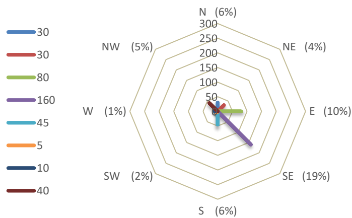
نمودار (۱۹) جهت، سرعت و درصد وزش باد در بهار (بیگلری، ۱۳۹۹).
