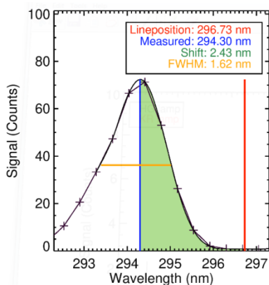
شکل ۱۵. تصحیح موقعیت مرکز طول موج متناسب با اندازه‌گیری‌های لامپ‌های کریپتون و جیوه
