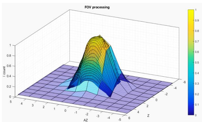
شکل ۱۱. میدان دید سه بعدی دهانه اپتیکی، در دو راستای زنیت و آزیموت و با دو حد تفکیک متفاوت ۰/۱ و ۱ درجه
