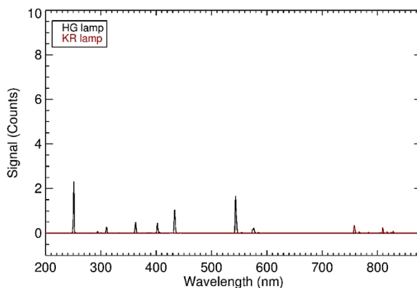
شکل ۱۴. موقعیت طول موج‌های مشخص لامپ‌های استاندارد کالیبراسیون کریپتون و جیوه
