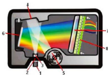
شکل ۲. ساختار درونی اسپکترورادایومتر. (۱) ارتباط با فیبر نوری، (۲) شکاف، (۳) فیلتر، (۴) آینه کولیماتور، (۵) شبکه انکساری، (۶) آینه متمرکز، (۷) لنز جمع کننده آشکارساز، (۸) آشکارساز CCD.
