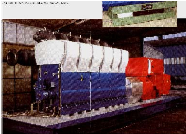
شکل ۴- نمایي از ماشین بخار مورد استفاده در نیروگاه خورشیدی شیراز
