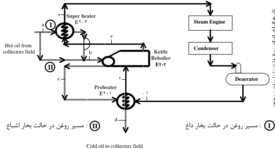
شکل ۳- نمایی شماتیک از سیکل بخار نیروگاه خورشیدی شیراز
