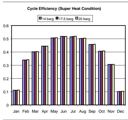
شکل ۱۷- تغییرات راندمان سیکل روغن در اثر تغییر فشار ورودی به ماشین بخار (حالت ارسال بخار داغ به ماشین بخار)
