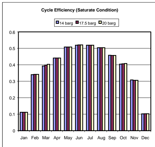
شکل ۱۸- تغییرات راندمان سیکل روغن در اثر تغییر فشار ورودی به ماشین بخار (حالت ارسال بخار اشباع به ماشین بخار)
