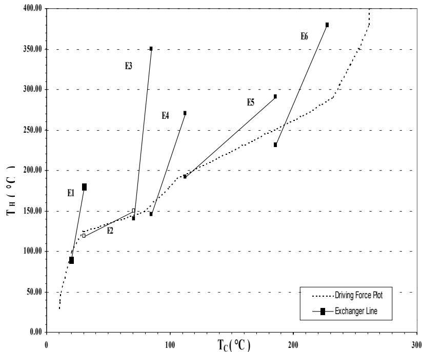
شکل ۶- منحنی نیروی رانش دمایی در \Delta T_{\min} = 58 \text{ } ^\circ\text{C} همراه با خطوط عملکرد مبدل‌های موجود
