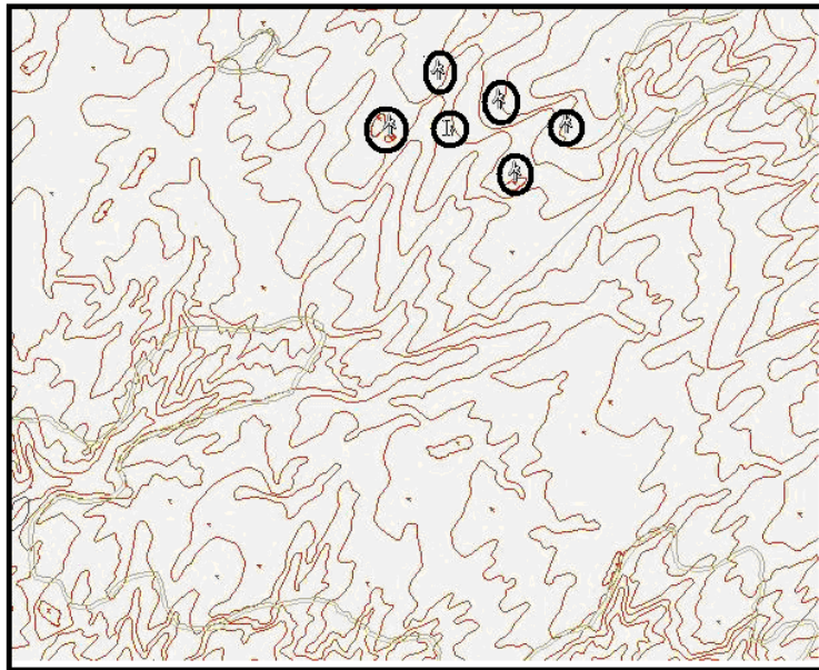
شکل ۱۰: چیدمان توربین های بادی 2MW
