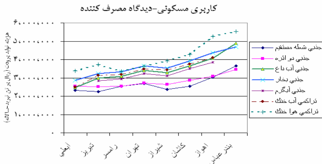
شکل (۱): تأثیر اقلیم بر هزینه تولید برودت در سیستم‌های سرمایشی با کاربری مسکونی و از دیدگاه مصرف کننده
