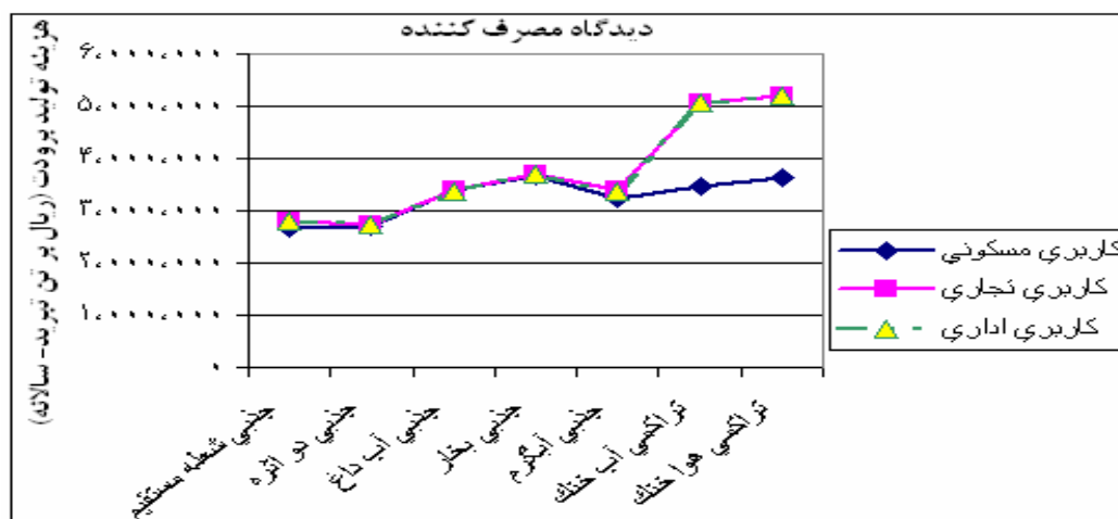
شکل (۲): تاثیر کاربری بر هزینه تولید برودت در سیستم‌های سرمایشی در شهر تهران و از دیدگاه مصرف کننده
