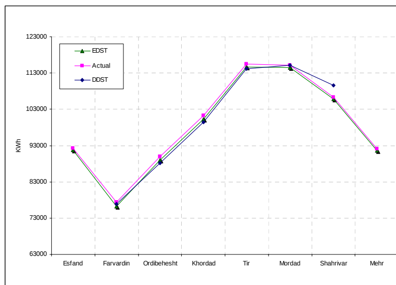
نمودار ۱۲- تغییرات متوسط مصرف روزانه برق در استان تهران ماههای مختلف و سناریوهای مختلف تغییر ساعت - ۶ ماه بهار و تابستان در سناریوهای DST و EDST یکسان است
