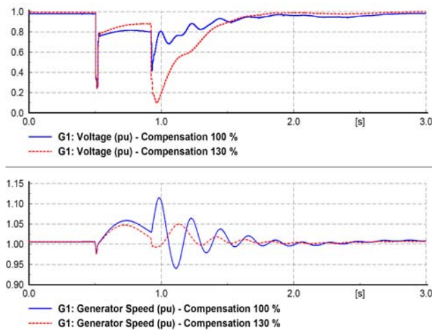
شکل(۸): نمودارهای ولتاژ و سرعت ژنراتور برای دو حالت جبران‌سازی توان راکتیو ۱۰۰ درصد و ۱۳۰ درصد و زمان عملکرد کلید ۲۰ میلی ثانیه
