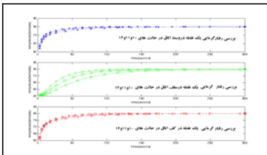
شکل ۶- بررسی اثر جنس covering در زمان گرمایش
