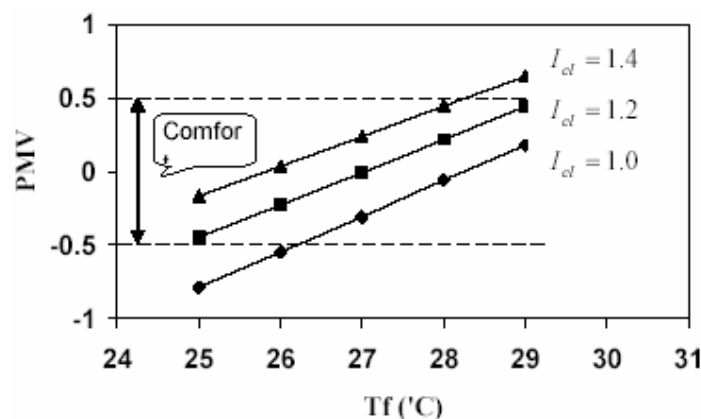
شکل ۵- احساس حرارتی افراد با تغییر میزان لباس، R_w = 4 (m^2 K/W) و \varepsilon = 0.9
