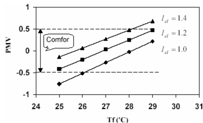
شکل ۶- احساس حرارتی افراد با تغییر میزان لباس، R_w = 4 (m^2 K/W) و \varepsilon = 0.95
