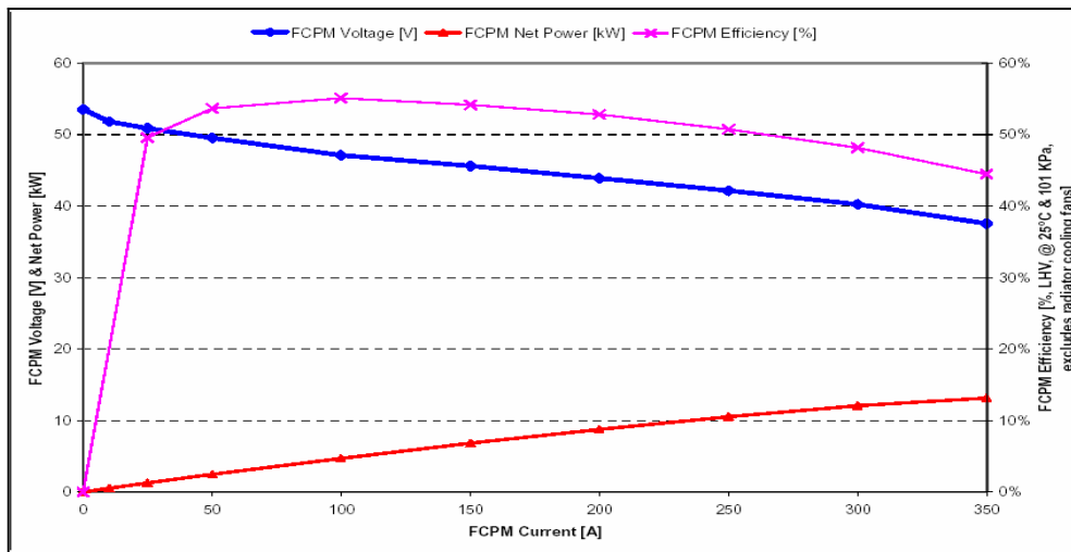
شکل (۱۹): نمودار زیر عملکرد نرمال پیل سوختی [۵]
