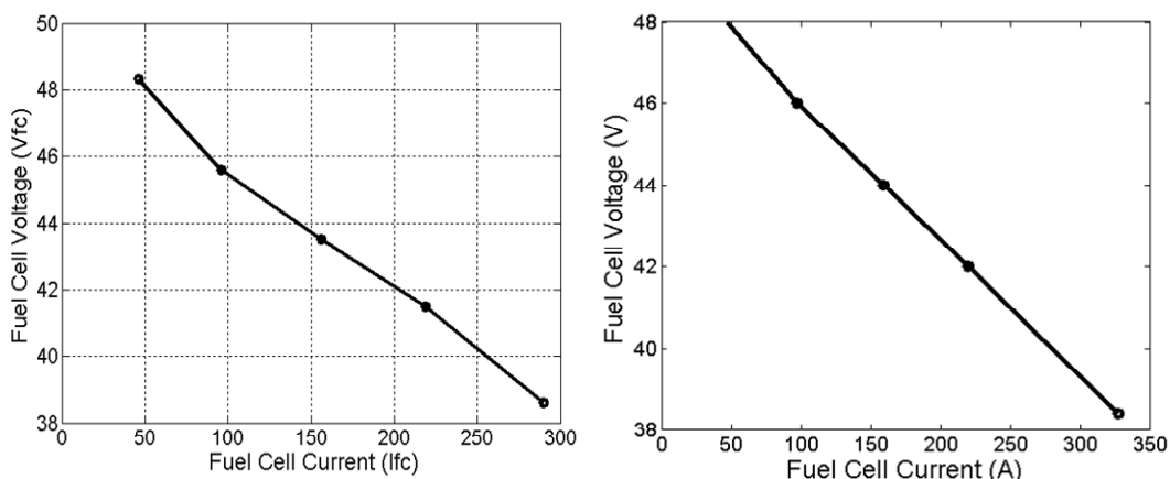
شکل (۲۲ و ۲۱): منحنی تغییرات ولتاژ پیل سوختی بر حسب جریان پیل سوختی برای هر دو پیل سوختی به شبکه سایت طالقان
