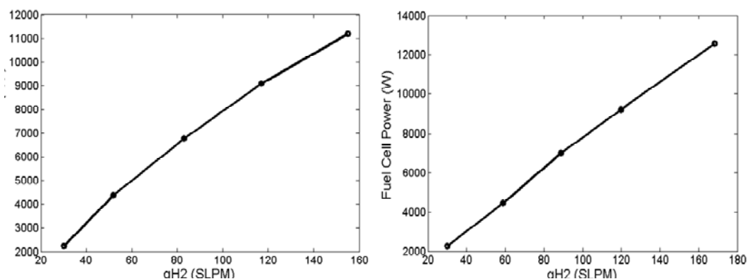
شکل (۲۴ و ۲۳): منحنی تغییرات توان پیل سوختی بر حسب تغییرات سوخت مصرفی برای هر دو پیل سوختی
