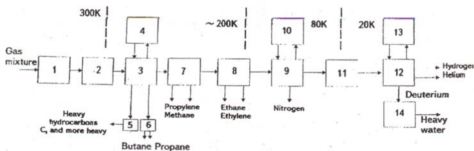
شکل ۲- شماتیک دستگاه سرمایه عمیق برای تولید مواد مختلف
