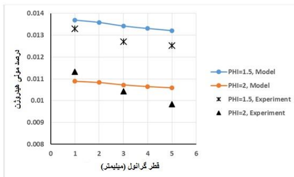
شکل ۱۱. تغییرات هیدروژن تولیدی در خروجی راکتور برای قطره‌های مختلف گرانول با نسبت هم‌ارزی‌های مختلف
