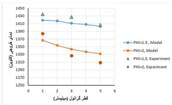
شکل ۱۰. تغییرات دما در خروجی راکتور برای قطره‌های مختلف گرانول با نسبت هم‌ارزی‌های مختلف
