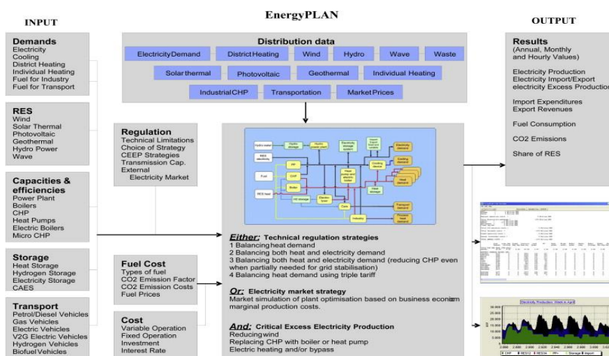
شکل ۲. ساختار مدل انرژی پلن [۱۵]
