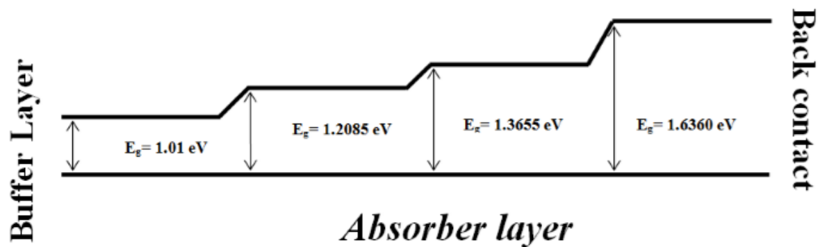
شکل ۲: پروفیل های باند شکاف جذاب سلول خورشیدی CIGS
