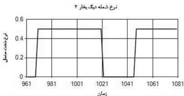
شکل ۱۲ ب) نمودار خروجی کنترلر خطی مشعل دیگ بخار (استراتژی پیشنهادی)
