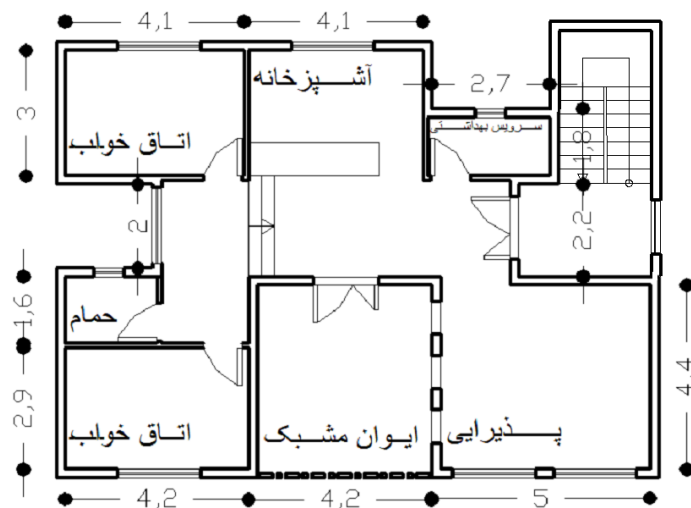
شکل 1) نقشه طبقات آپارتمان مسکونی 4 طبقه بر روی پیلوت در شهرستان بابلسر
