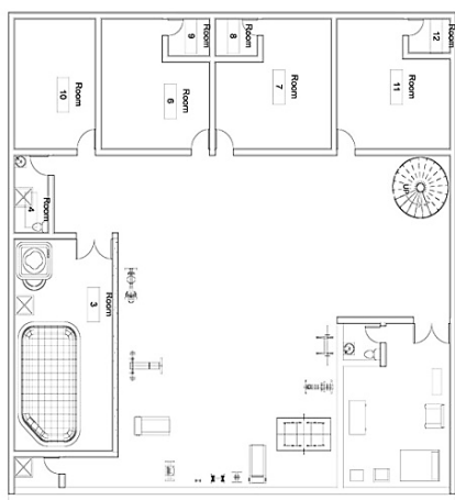
شکل ۱۰. پلان همکف واحد بدون گودال باغچه
