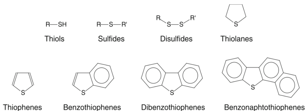
شکل ۱. انواع مختلفی از ترکیبات آلی گوگردی در نفت خام (جوادلی و کلرک، ۲۰۱۱).
