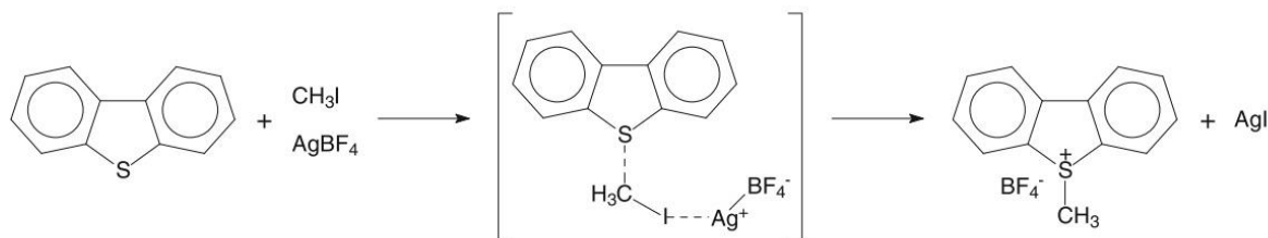
شکل ۷. گوگردزدایی مبتنی بر آلکیلایسیون گوگرد (سانگ، ۲۰۱۳).
