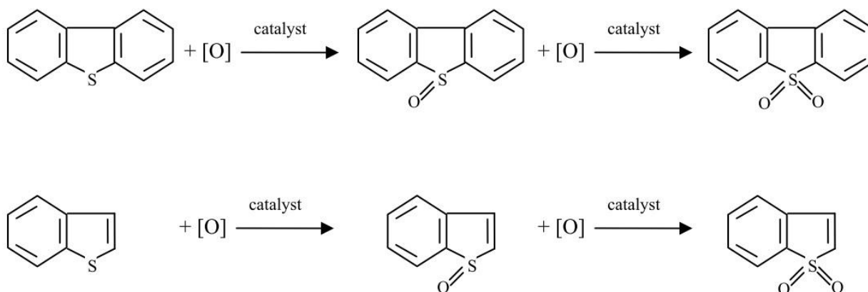
شکل ۵. واکنش‌های کلی BT و DBT در فرایند ODS (ساتبا، ۲۰۱۳).
