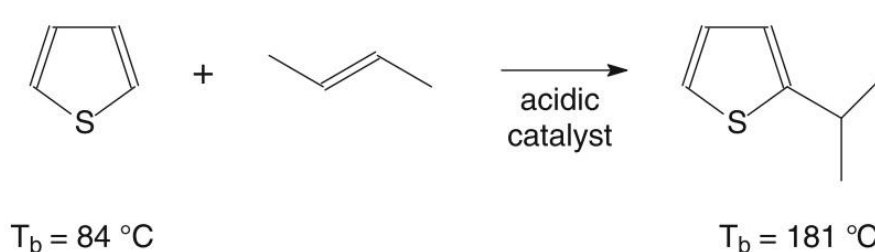
شکل ۶. گوگردزدایی مبتنی بر آلکیل‌اسیون از طریق آلکیل‌دار تیوفن با استفاده از ۲-پنتن جهت.
