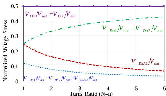
شکل ۵: تنش‌های ولتاژ نرمالیزه شده دو سر نیمه هادی‌ها.
