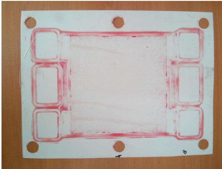
شکل ۴. تاثیر عدم یکنواختی فشار بر روی صفحه حساس
