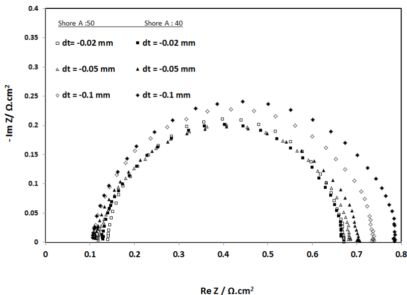
شکل ۳. نمودارهای مختلف EIS ناشی از تاثیر تغییر ضخامت و سختی واشرهای گاز
