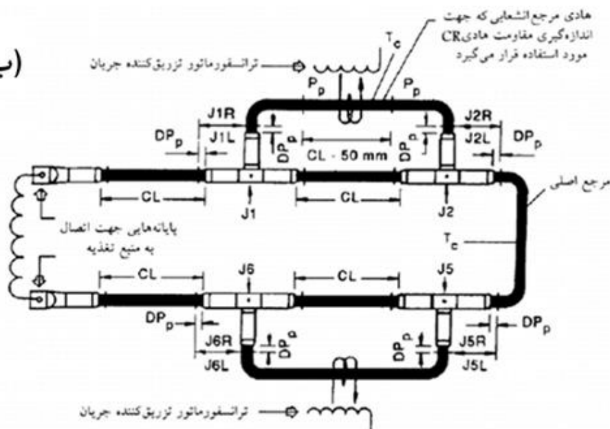
شکل ۳. مدار الکتریکی آزمون سیکل جریان/حرارتی برای بررسی تغییرات مقاومت الکتریکی/دمای اتصالات (الف) کششی (کلاس A) و (ب) غیر کششی (کلاس B) [۱۳]
