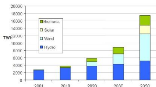
شکل (۱) پیش بینی میزان تامین انرژی الکتریکی های تجدید پذیر در جهان تا سال ۲۰۵۰ [۱۱]
