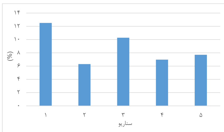
شکل ۷. درصد انحراف معیار تغییرات لاین پک همه لوله‌های گاز
